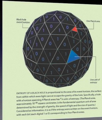
Bekenstein Hawking
