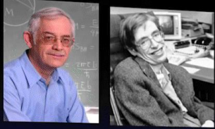
Bekenstein Hawking
